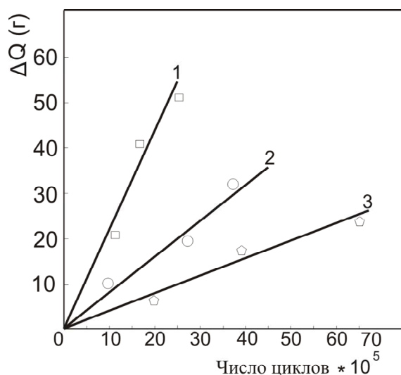
Рисунок 2 - Износ образцов, вырезанных из прокатных валков
