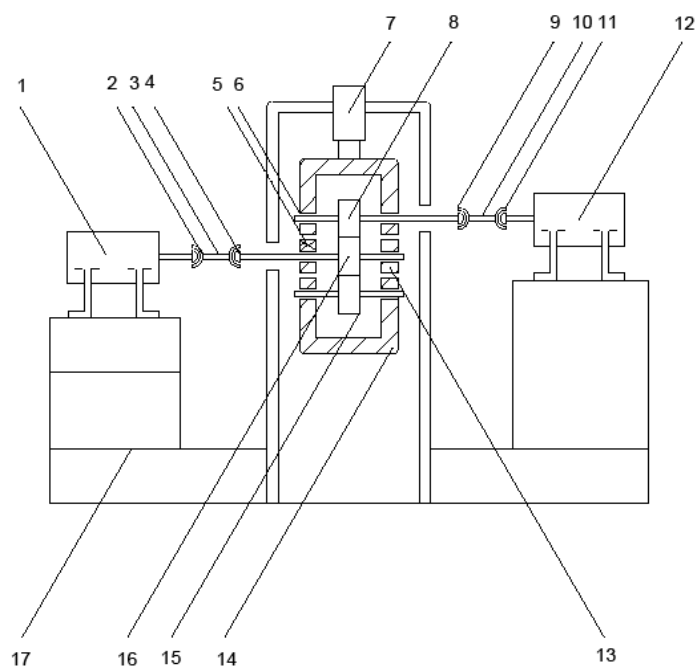
Рисунок 1 - Принципиальная схема роликовой испытательной машины
